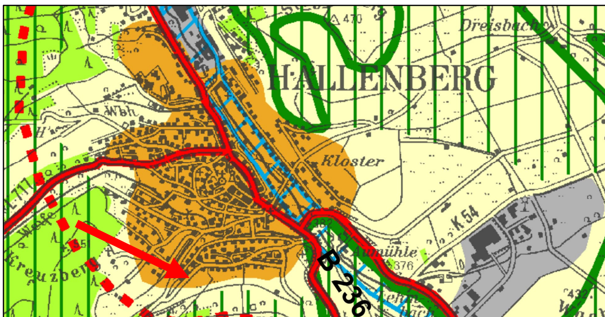
Abbildung 3: Ausschnitt aus dem Regionalplan Arnsberg (2012)
