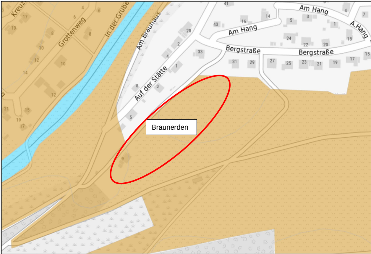
Abbildung 13: Bodentypen im Eingriffsgebiet (Quelle: Geologischer Dienst NRW)
