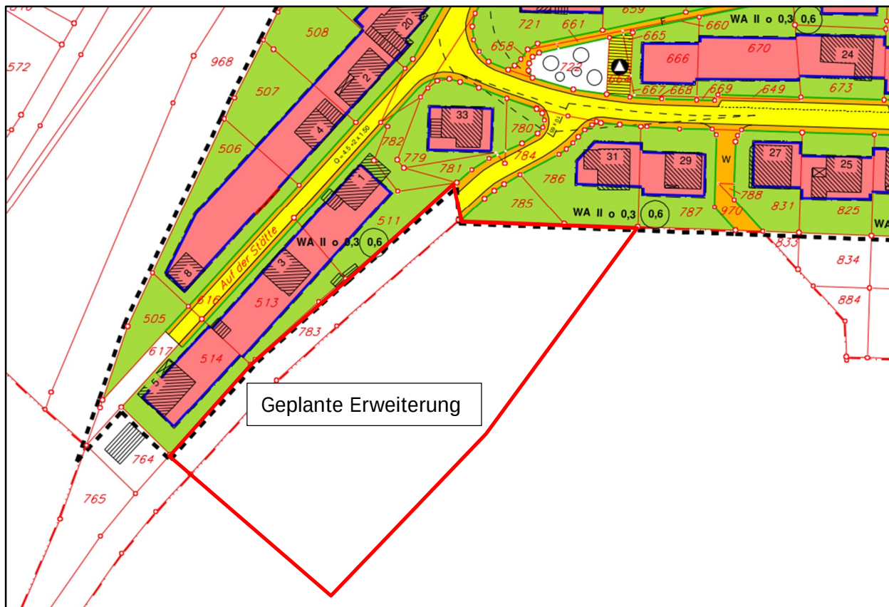
Abbildung 5: Bebauungsplan Nr. 2 „Langeloh - 5. Änderung (Ausschnitt)
